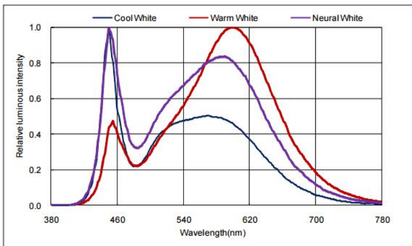
Radiation diagram 辐射图特性曲线
